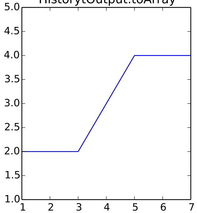
HistoryOutput.toArray
